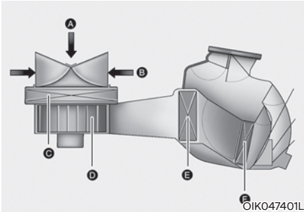
[A] : Vanjski zrak, [B] : Recirkulirani zrak [C] : Filtar zraka klima-uređaja, [D] : Ventilator [E] : Isparivač, [F] : Grijač
